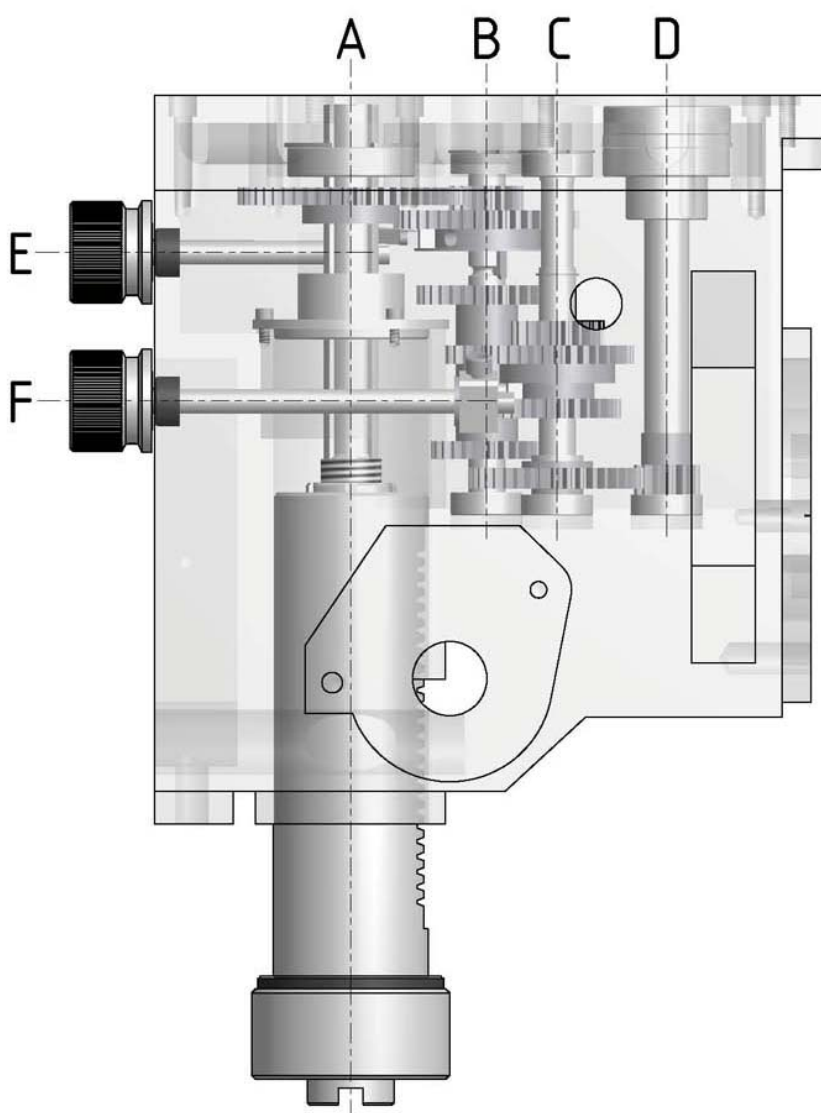
Abb.8-1: Fräskopf 1 von 6 - Milling head 1 von 6
