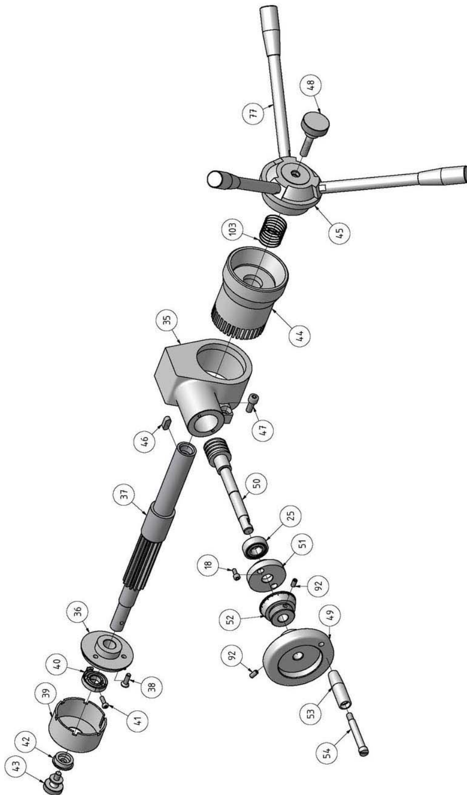
Abb.8-5: Fräskopf 5 von 6 - Milling head 5 von 6
