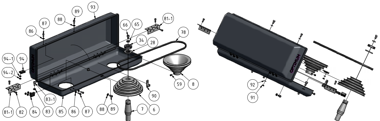
Abb.1-2: Keilriemenscheiben B16H - Pulleys B16H
