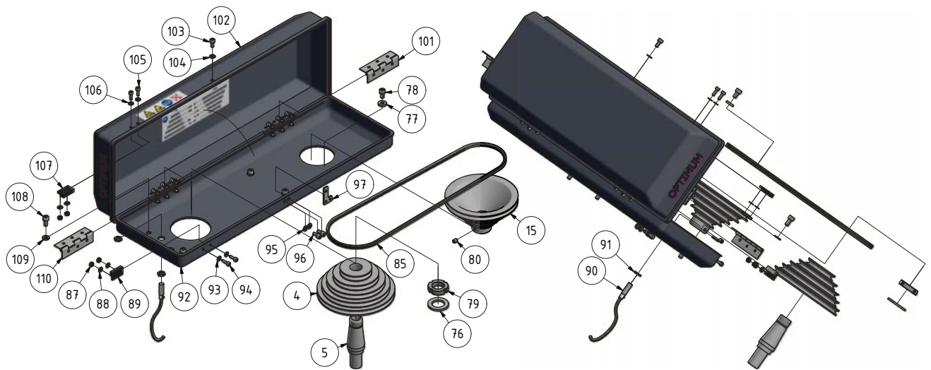
Abb.1-5: Keilriemenscheiben - Pulleys
