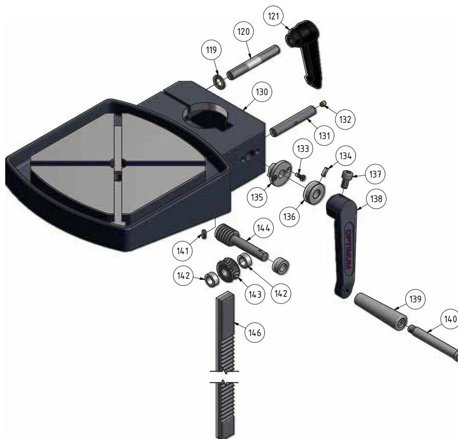
Abb.1-7: Bohrtisch - Drilling table
